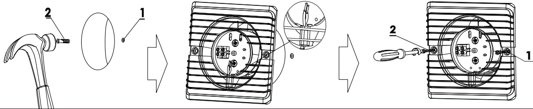
Instalowanie wentylatora/ Fan installation/ Lüftereinbau
