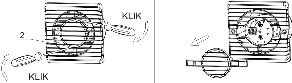
Demontaż kratki/ Grill disassembly/ Demontage des Gitters
